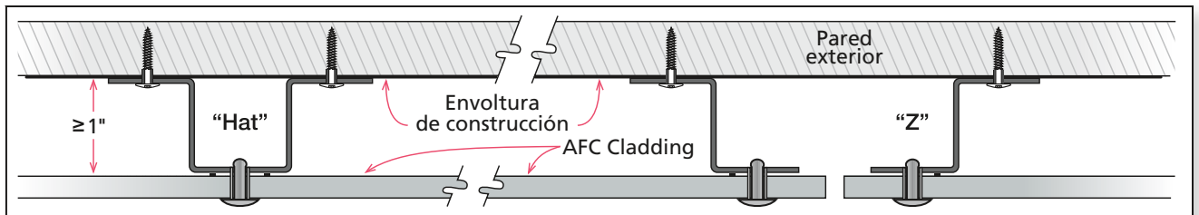
FIG. J — Canales "Hat" o "Z" y junta vertical. (Canales G90 y recubiertos "Z" con pintura de polvo, ofrecidos por AFCC).
