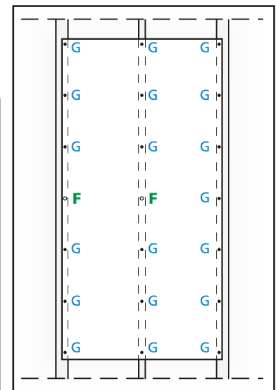
▼ FIG. F — Instalación vertical en perfiles verticales.
