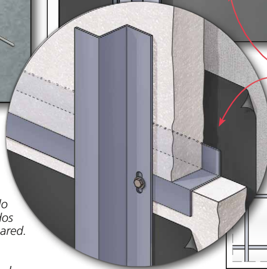
FIG. J — Canales "Hat" o "Z" y junta vertical. (Canales G90 y recubiertos "Z" con pintura de polvo, ofrecidos por AFCC).
